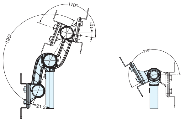
KA-TLG2-100 (Dual Axis)
